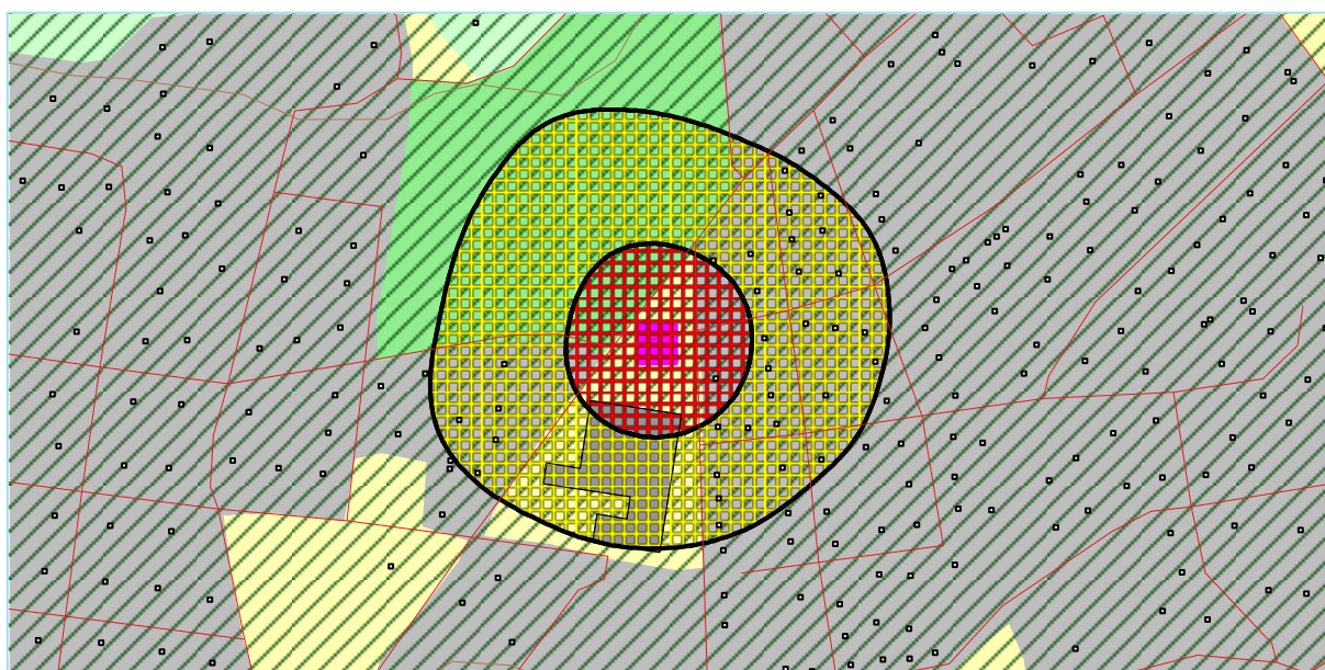
Figur 9-2. Støysoner for Hamar helikopterlass sykehuset. Målestokk 1:5 000.
