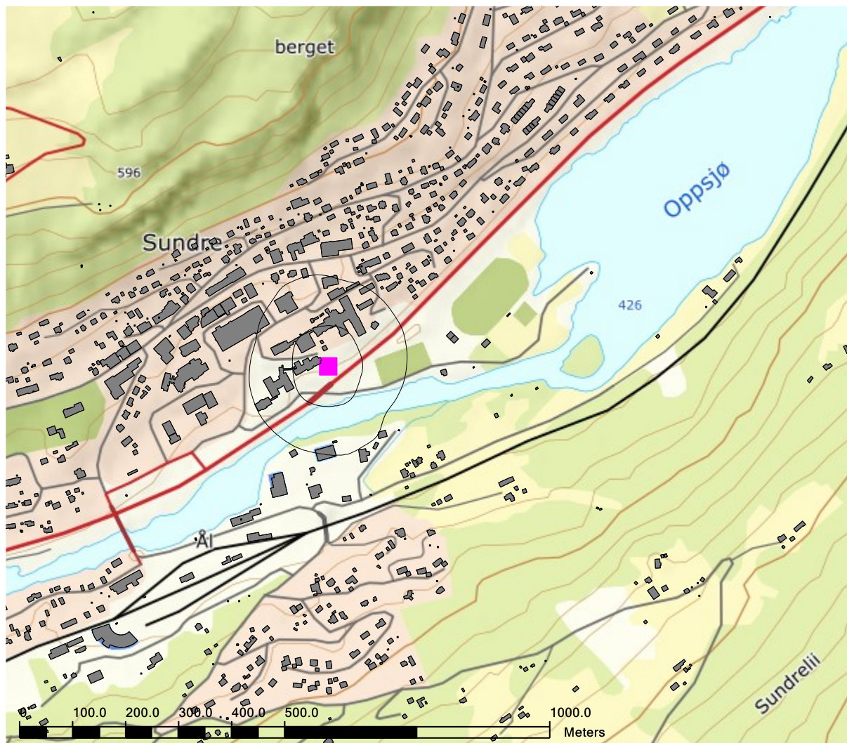
Figur 8-3. L_{5AS} 80 og 90dBA for prognosen. M 1:10 000.
