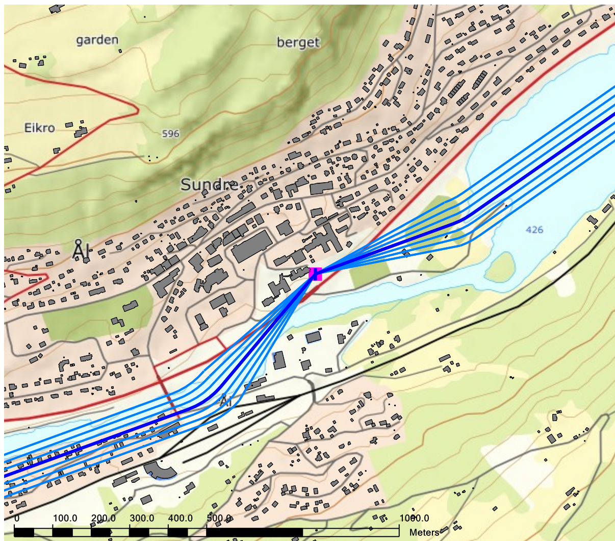
Figur 7-1. Traséer for inn- og utflyging, inkludert spredtraséer.
