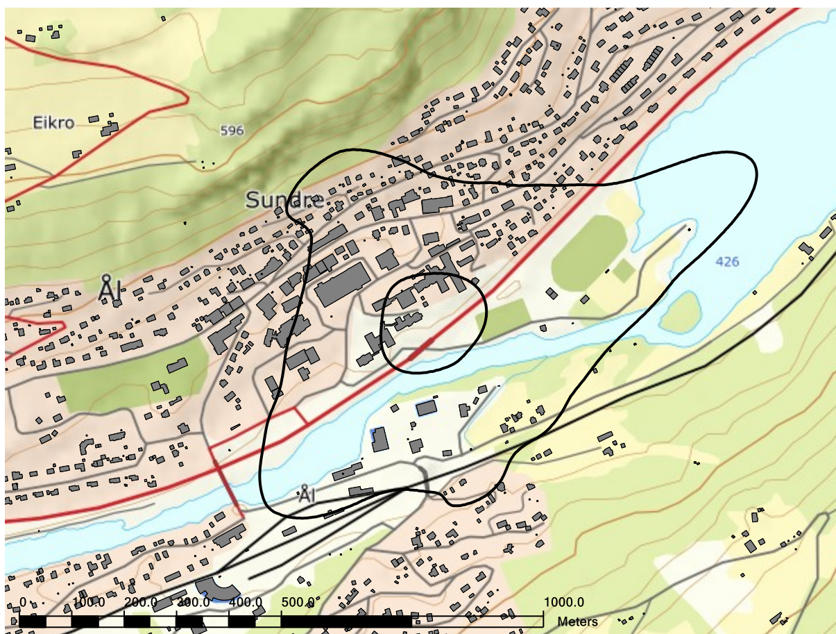
Figur 8-1. L_{den} 52 og 62dBA for 2021. M 1:10 000.
