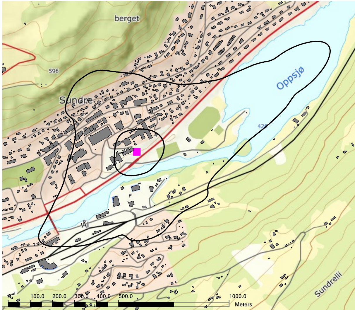
Figur 8-2. L_{den} 52 og 62dBA for prognosen. M 1:10 000.
