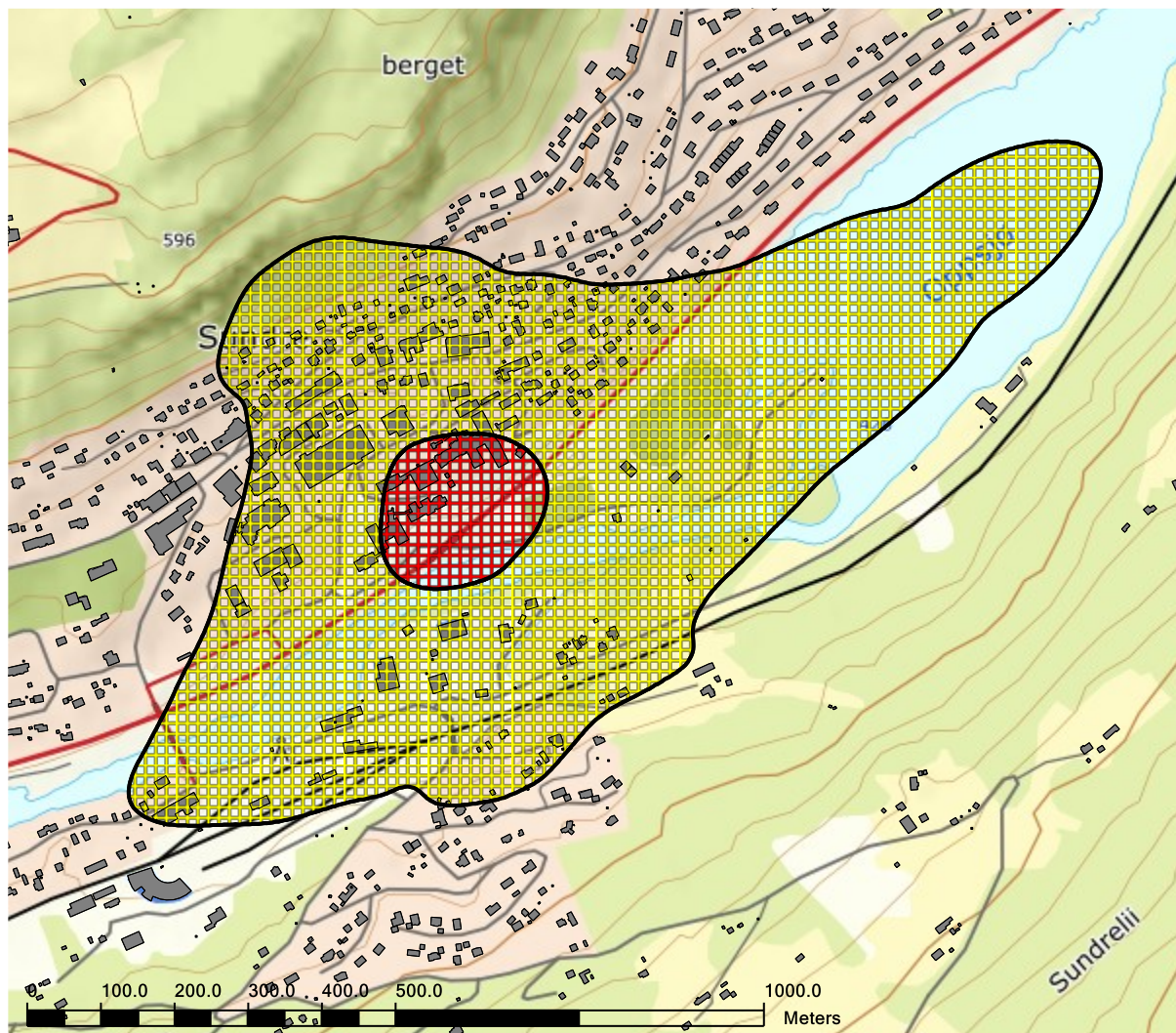
Figur 8-4. Støysonkart for Ål helikopterplass. M 1:10 000.
